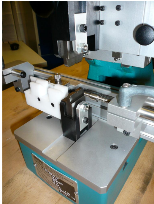
Werkzeug offen
