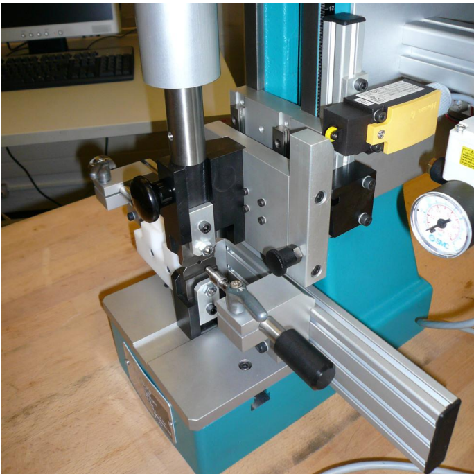
Werkzeug geschlossen
